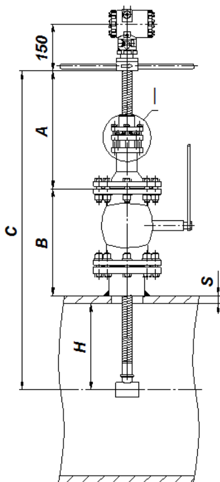
Рисунок 2.4 Вычисление глубины погружения датчика
